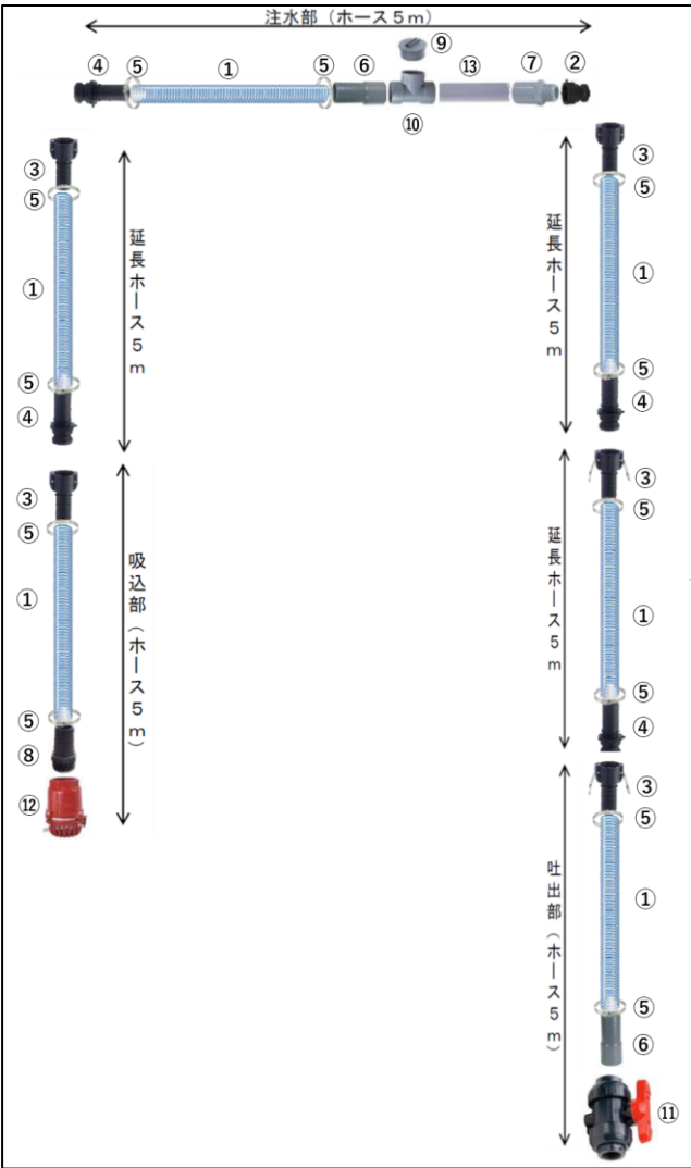
貸し出し装置の模式図
